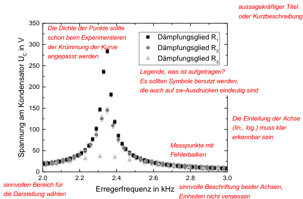
Abbildung 1: Amplitudenresonanzkurve im Reihenschwingkreis mit variierender Dämpfung
